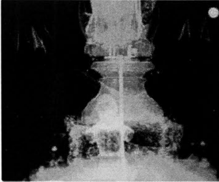
Figura 5. Anclaje de la escultura a una pletina con cuatro tornillos y un perno que llega hasta la base del fanal. Estudio de rayos X. Archivo CNCR. (C. Correa, 2018).
