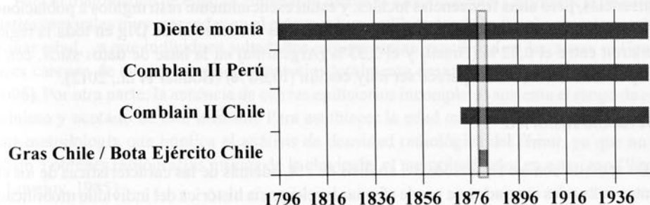
Figura 27. Concentración de carbono 14 en las muestras. En gris oscuro se señalan las probabilidades estadísticas de la localización temporal del individuo, considerando el margen de error.
