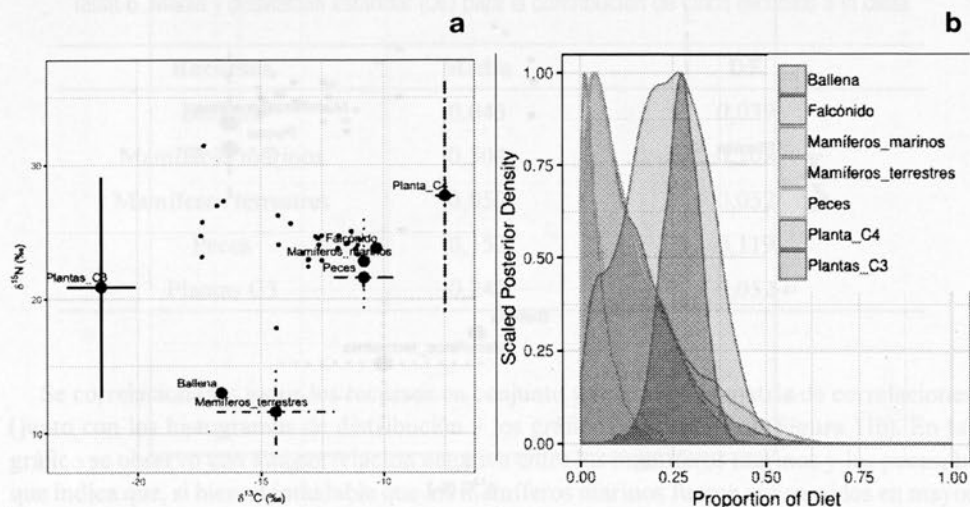
Figura 9. a. Dispersión de individuos (puntos pequeños) y de recursos (puntos grandes). Las líneas representan la desviación estándar de los recursos. Se consideró fraccionamiento de 2,6‰ en 13C y de 3,1‰ en 15N. b. Distribución posterior de la contribución de siete recursos a la dieta.
