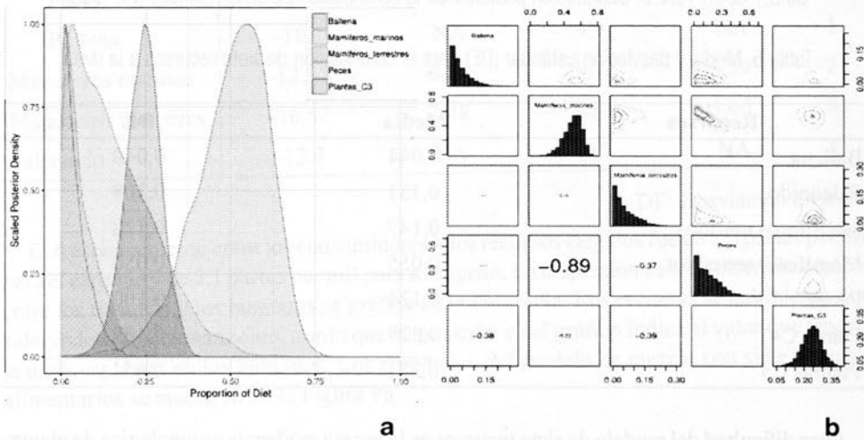
Figura 11. a. Distribución posterior de la contribución de cinco recursos a la dieta. b. Matriz de correlaciones. La línea diagonal muestra el histograma de distribución para cada recurso, la mitad superior la
