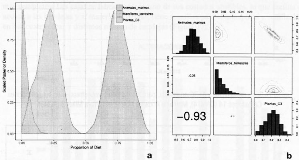
Figura 13. a. Distribución posterior de la contribución de tres conjuntos de recursos a la dieta. b. Matriz de correlaciones. La línea diagonal muestra el histograma de distribución para cada recurso, la mitad superior la matriz de contornos y la mitad inferior la matriz de correlaciones. Destaca la alta correlación negativa entre animales marinos y plantas C3.
