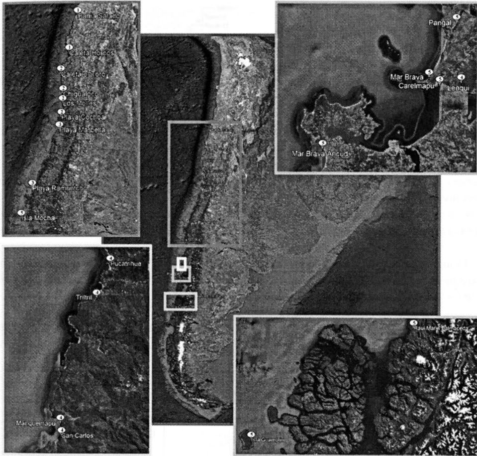
Figura 2. Poblaciones de Orchestoidea tuberculata analizadas en el estudio, indicando los grupos a los que pertenecen (grupos N°1 a 5) .
