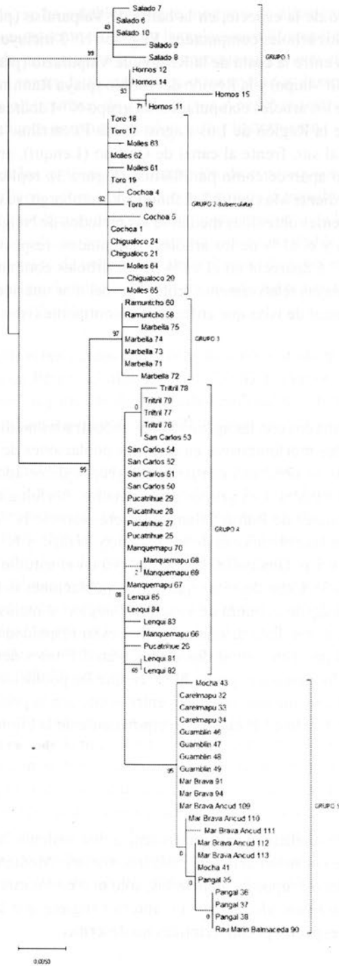
Figura 3. Filogenia reconstruida mediante el método Maximum Likelihood y el modelo de Tamura-Nei. Se muestra el árbol con el más alto valor de verosimilitud (-1181,93).
