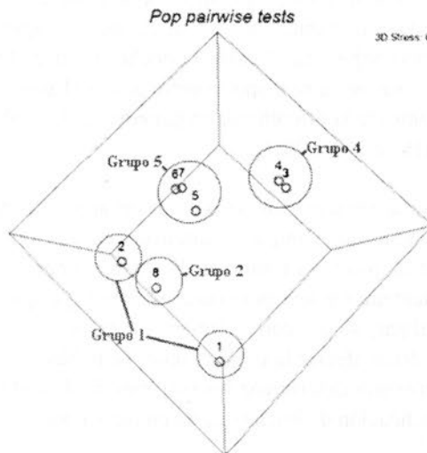
Figura 1. Representación espacial tridimensional de las diferencias en el tamaño de los rasgos morfológicos de distintas poblaciones (según Pérez-Schultheiss et al. , 2018) y asignación de las poblaciones a los grupos detectados mediante ABGD. Poblaciones: 1, Bahía Salado; 2, Caleta Hornos; 3, Pucatrihue; 4, Triltil; 5, Pangal; 6, Carelmapu; 7, Isla Guablín y 8, Playa Cochoa.
