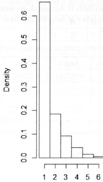
Figura 3. Distribución de probabilidad a posteriori de los cluster (K) o poblaciones de Arbacia spatuligera a lo largo de la cadena de Markov Monte Carlo (MCMC).
