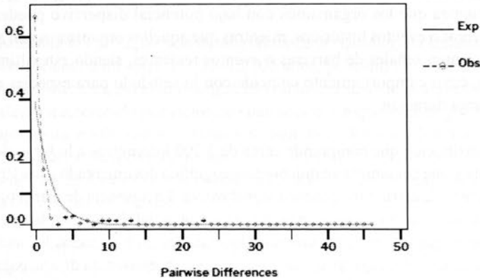
Figura 4. Distribución de desajuste entre pares de secuencias de Arbacia spatuligera del PSE.
