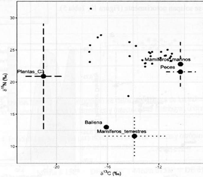
Figura 10. Dispersión de individuos (puntos pequeños) y de los cinco recursos (puntos grandes). Las líneas representan la desviación estándar de los recursos. Se consideró fraccionamiento de 2,6‰ en ^{13}\text{C} y de 3,1‰ en ^{15}\text{N} .
