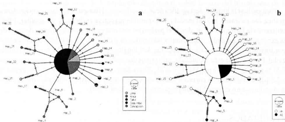
Figura 2. Red de haplotipos de Arbacia spatuligera en el PSE. a. Agrupadas por provincias biogeográficas (PP: Provincia Peruviiana, AI: Área Intermedia) y b. por poblaciones muestreadas a lo largo del PSE.
